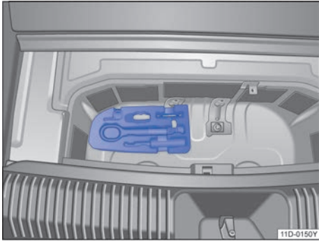
图 149 随车工具布置
