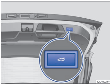
图 52 在打开的行李厢盖内：电动关闭行李厢盖的按钮
