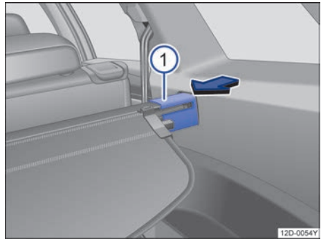
图 137 行李厢内：拆卸行李厢盖板
