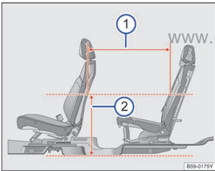
图 79 前排座椅和第二排座椅的座间距
