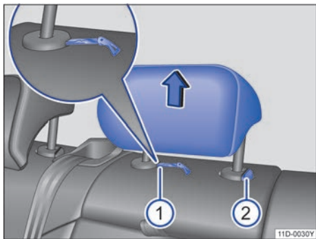
图 75 拆卸和安装后排头枕
