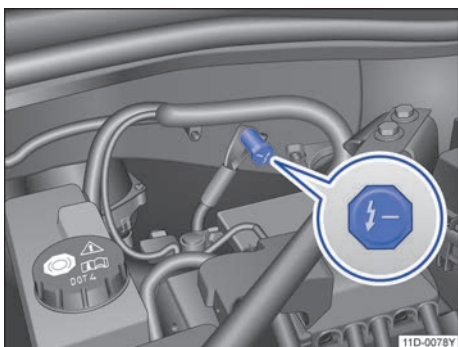
图 157 车身上的负极（接地点）
