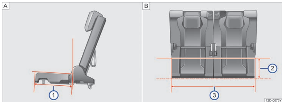
图 84 第三排座椅座宽和坐垫深
