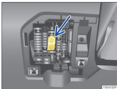
图 155 救援用保险丝
