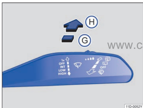
图 93 后风窗刮水器操纵杆操作位置
