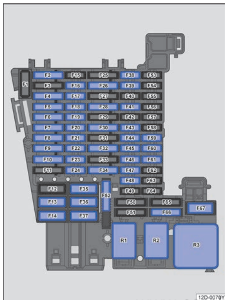
图 154 保险丝位置示意图
