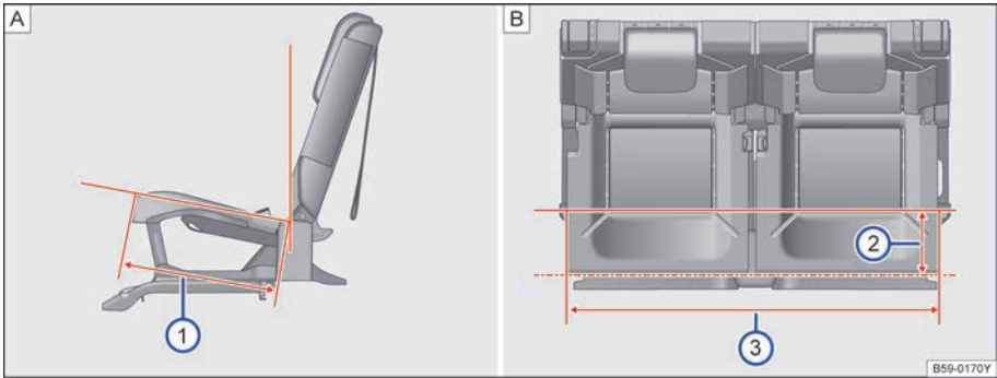
图 78 第三排座椅座宽和坐垫深
