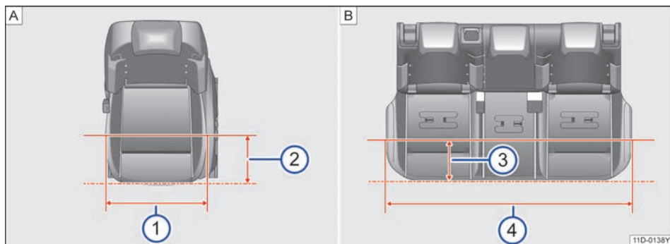
图 69 座椅座宽
