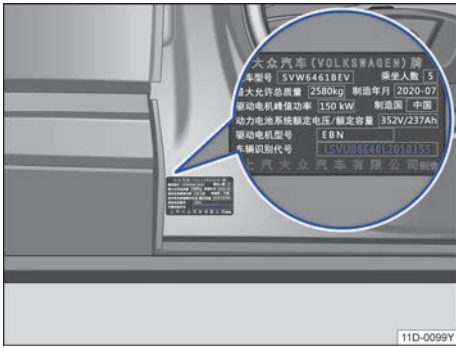
图 156 B 柱下方整车产品标牌
