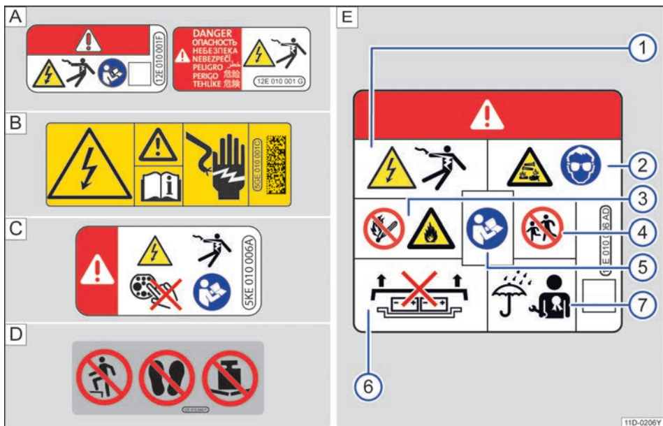
图 124 部分车型警告牌（示意图）：A. 高压组件 B. 高压电普通警告牌 C. 充电口高压警示标签 D. E. 高压电池上的警告牌
