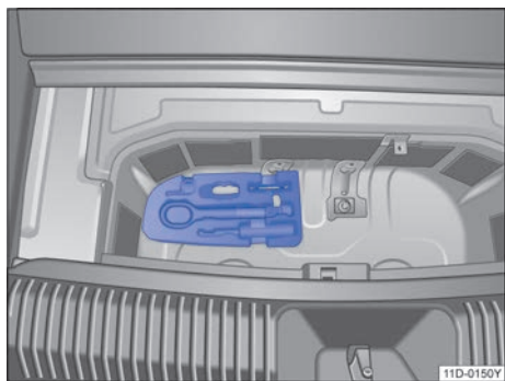
图 132 随车工具布置
