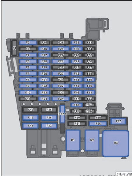
图 137 保险丝位置示意图
