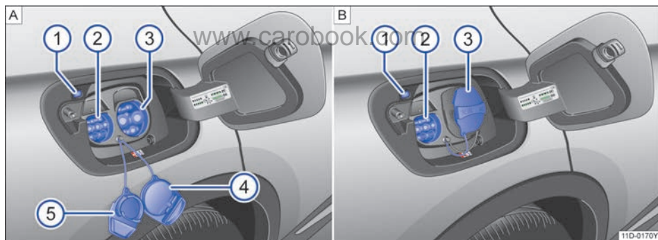
图 128 A 充电插口 B 充电口保护盖使用说明
